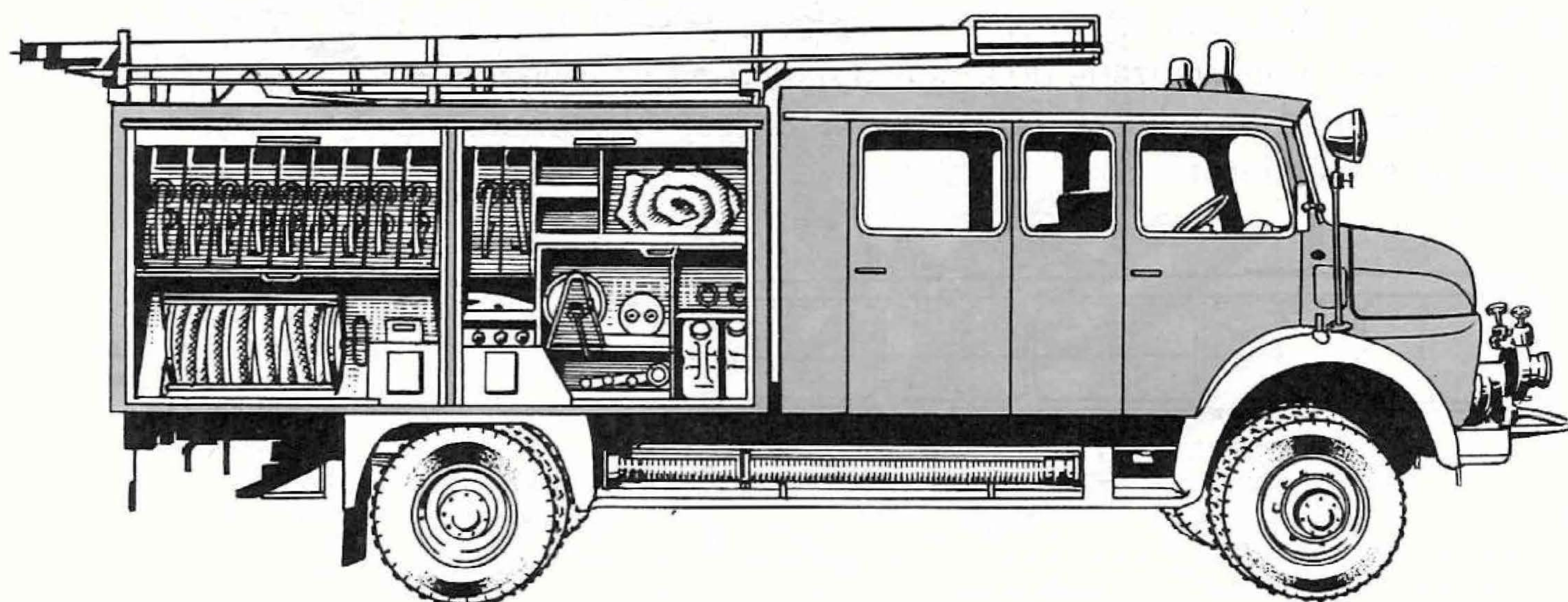
Rys. 4.17 Samochód gaśniczy
